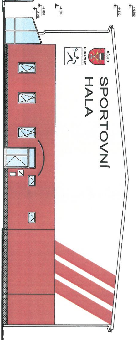
POHLED JIŽNÍ
