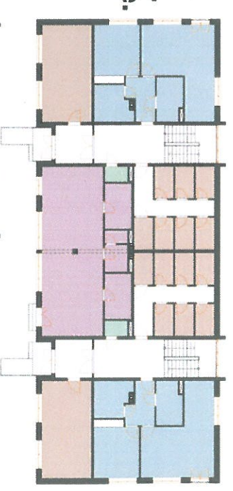
PŮDORYS SUTERÉN
